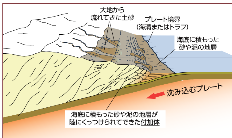
図 付加体の模式図
