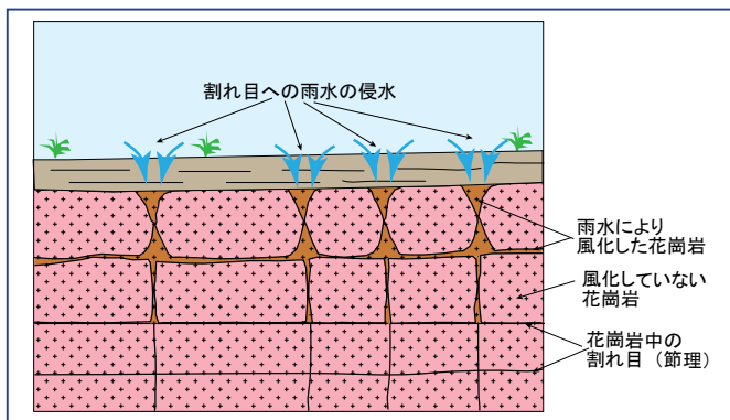
図1：花崗岩類の風化の模式図
