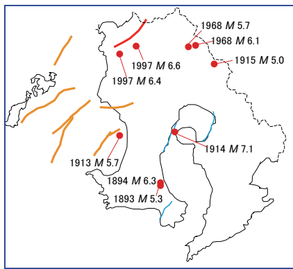
図2：1885年～2014年までに鹿児島県内で発生したM5以上の地震の分布図
