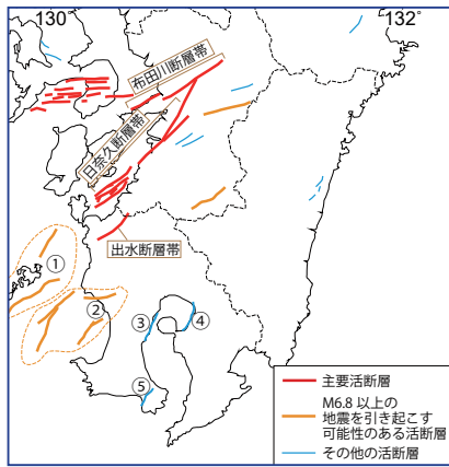
図1：九州中南部の活断層分布図
