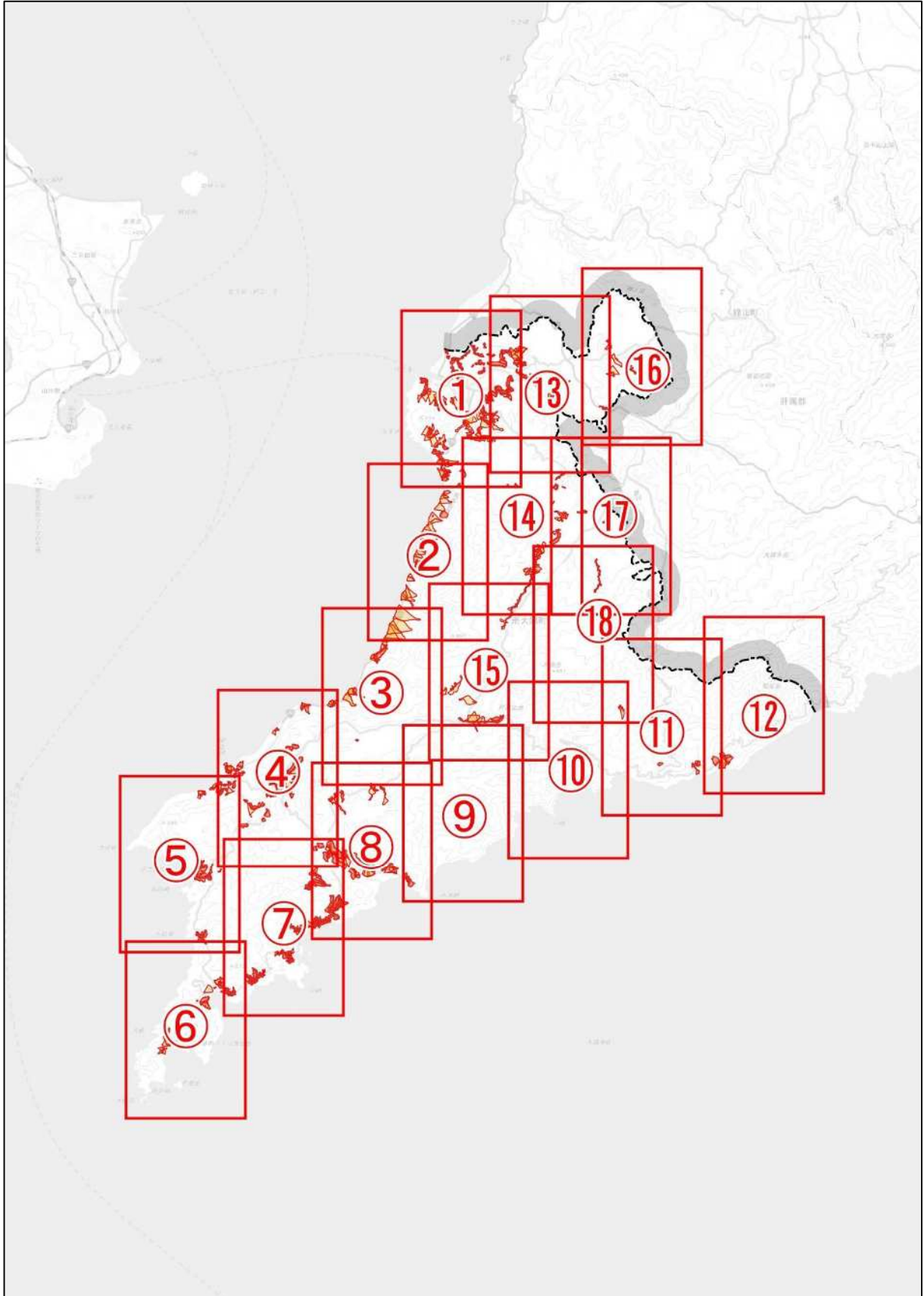
2-7 土砂災害警戒区域図
